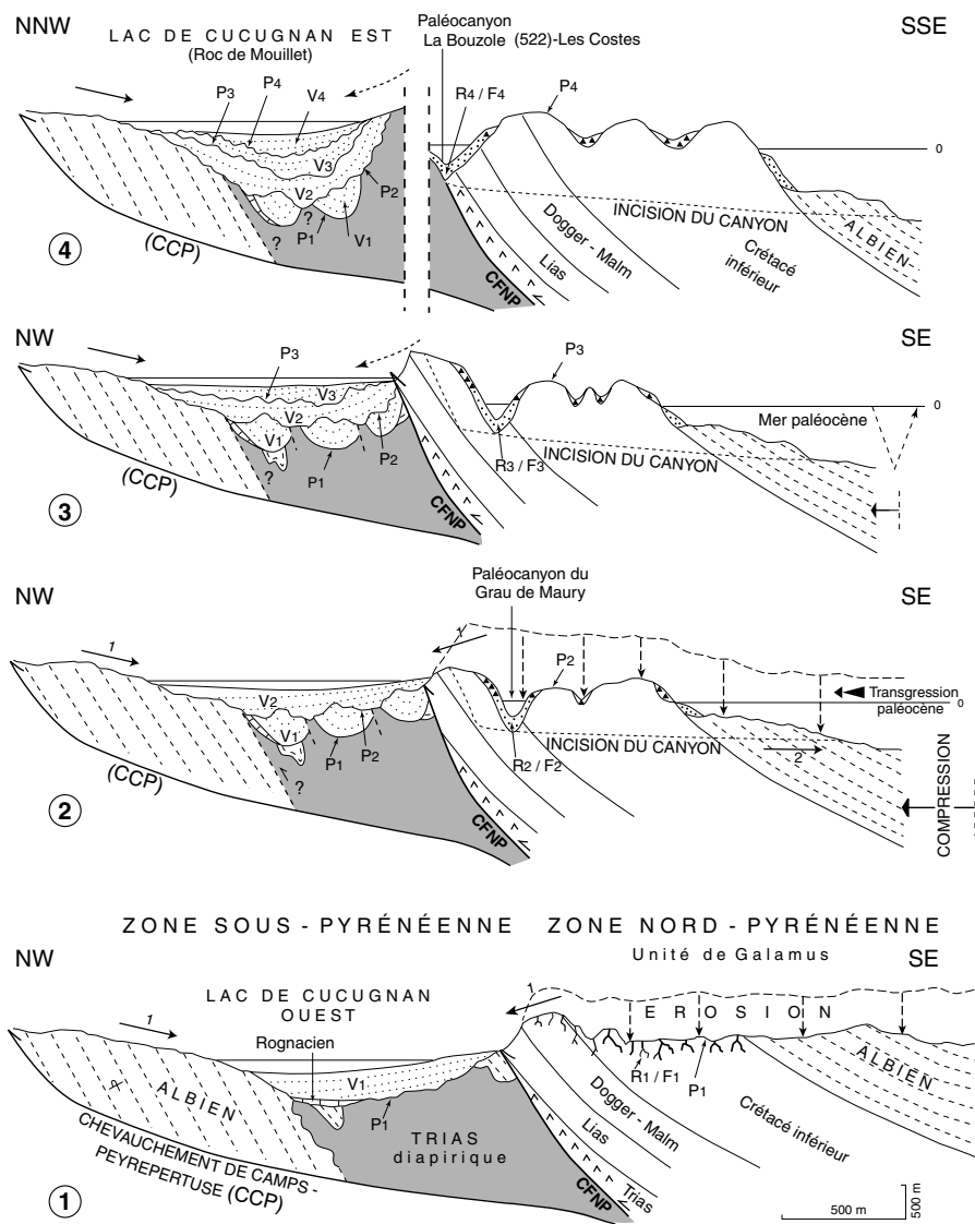
Fig. 12. Coupes palinspastiques reconstituant l'évolution tecto-sédimentaire et géomorphologique de la région de Cucugnan au Dano-Sélandien. Commentaire détaillé dans le texte.
