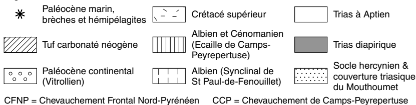
Fig. 2. Schéma structural simplifié de la région de Cucugnan. D'après les cartes géologiques à 1/50.000 de Tuchan (Berger et al. 1997) et Rivesaltes (Fontelles et al. 1993) modifiées.
