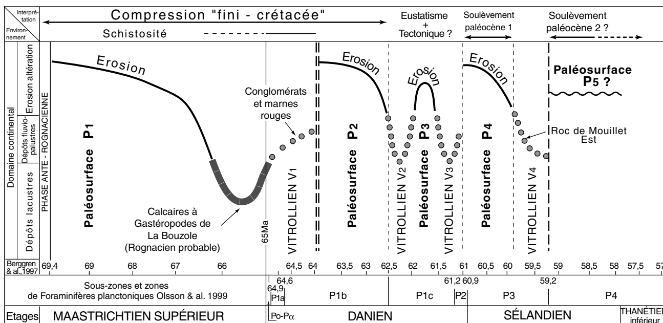
Fig. 13. Chronodiagramme synthétique sur les principaux événements et environnements de dépôt enregistrés dans la région de Cucugnan-Nord (Zone Sous-Pyrénéenne) au Crétacé terminal et au Dano-Sélandien. Commentaire détaillé dans le texte.
