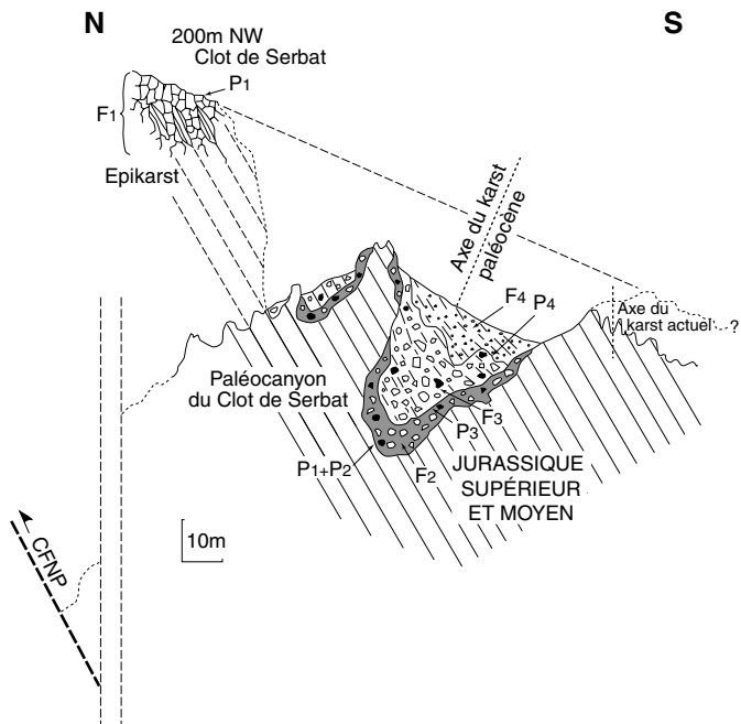
Fig. 6. Reconstitution schématique de la superposition des corps bréchiques et des paléosurfaces karstiques correspondantes dans le paléocanyon du Clot de Serbat.
